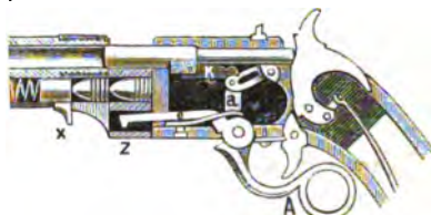
Č. 1691. Americká opakovačí bambitka z r. 1854.
